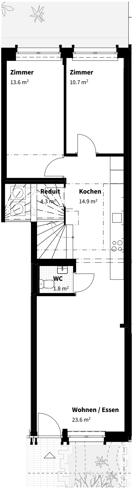
Wohnungsgrundriss
